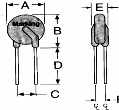
FRX 110-90F ~ FRX 375-90F Lead Size : 20AWG Φ 0.81 mm Diameter
